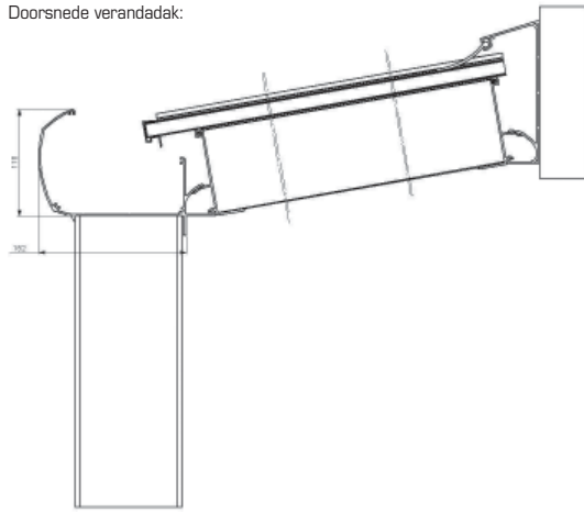
Doorsnede verandadak:
