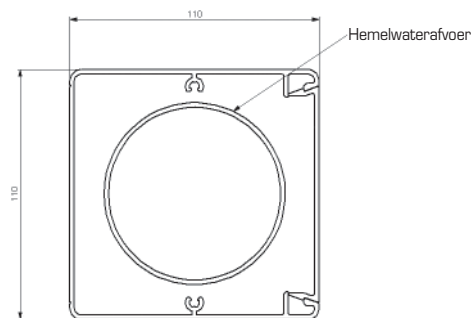
Doorsnede van standaard staander van bovenaf gezien:
